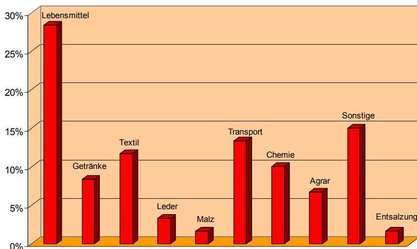
In Task 33/IV erfasste solare Prozesswärmeanlagen (Stand Oktober 2005): Verteilung auf Branchen
